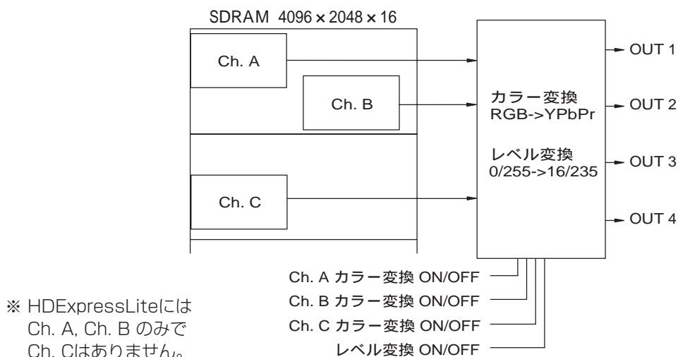
図1-1 表示チャンネルとカラー変換の対応
