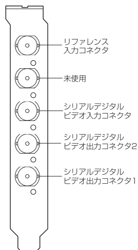
図2-4 HDEExpressLiteコネクタ配置図
