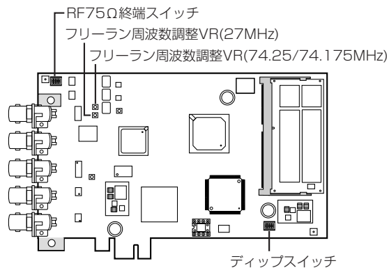
図2-2 HDEExpressLiteカード外観
