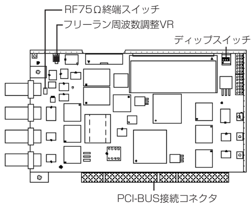
図2-1 HD64PCI/HD64DX4カード外観
