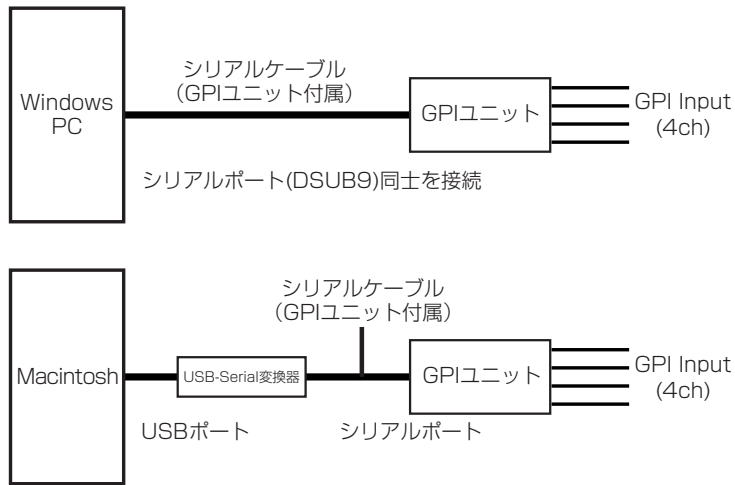
図4-12-11 GPIユニットの接続方法
