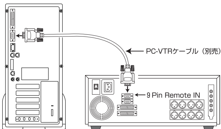
図4-12-9 VTR機器の接続
