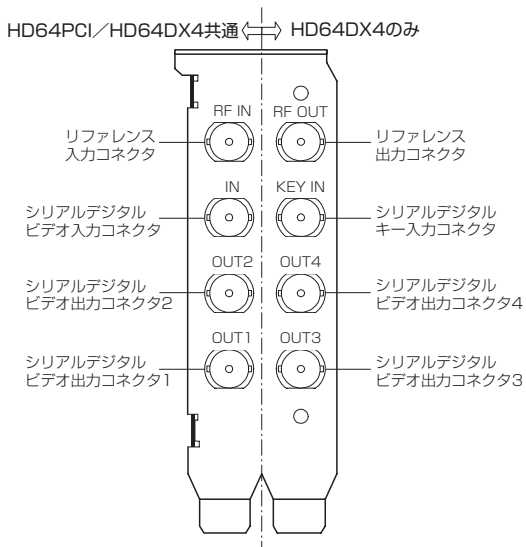
図2-3 HD64PCI/HD64DX4コネクタ配置図
