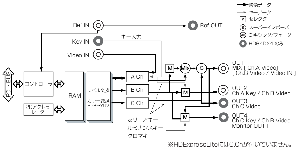
図1-3 入出力系統の概略
